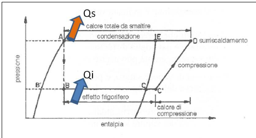
Figura 22 - Ciclo frigorifero sul diagramma pressione-entalpia
