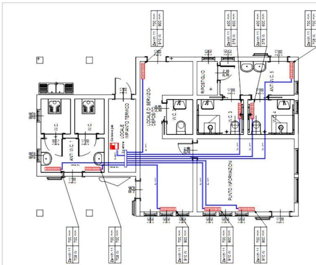
Figura 98 - Esempio di schema di distribuzione
