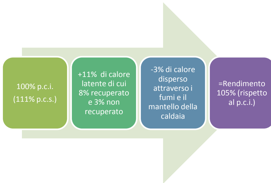
Figura 12 – Rendimento di una caldaia a condensazione alimentata a metano
