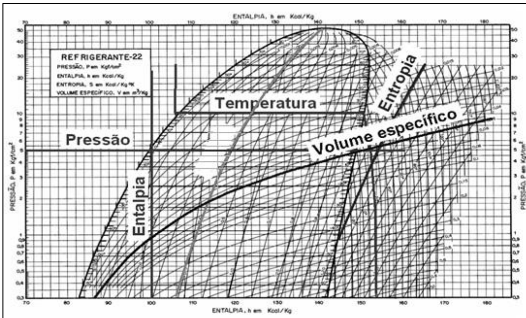
Figura 21 - Diagramma di Mollier per il Freon R22
