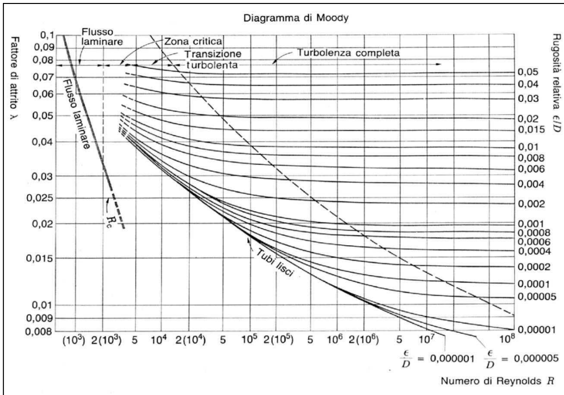
Figura 26 - Diagramma di Moody
