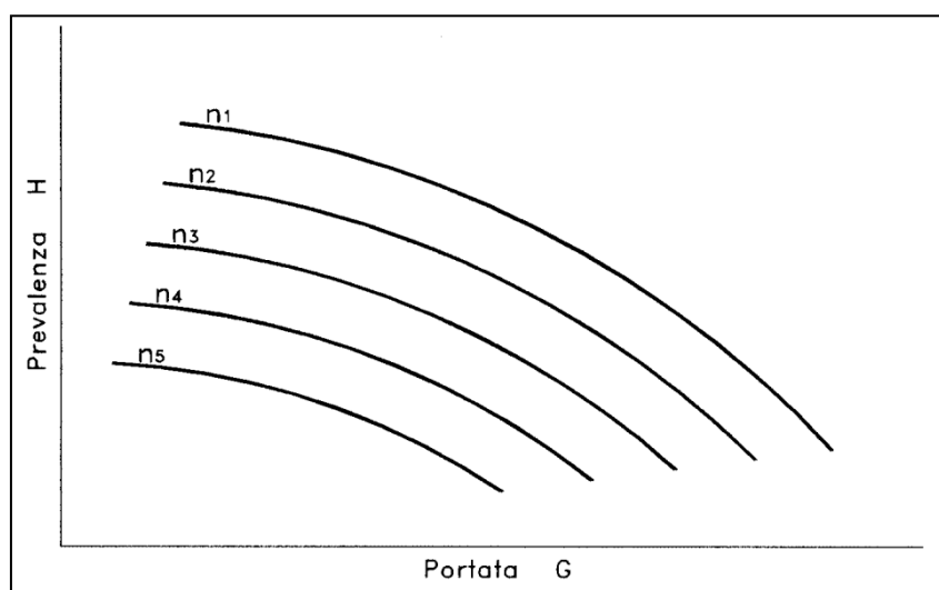
Figura 89 - Curva caratteristica di una elettropompa
