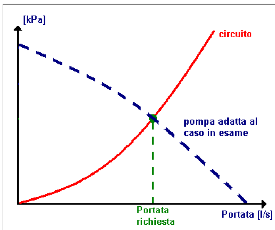
Figura 93 - Scelta della curva della pompa
