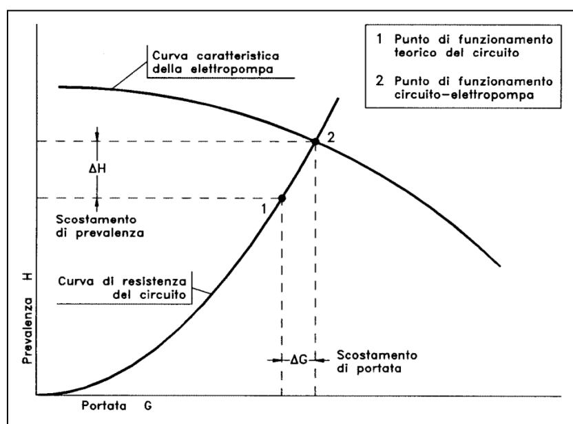
Figura 92 - Caratteristica circuito-pompa
