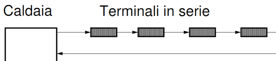
Figura 27 - Rete di distribuzione monotubo
