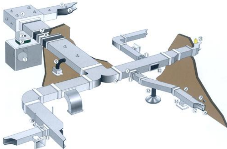
Figura 69 - Una distribuzione aeraulica
