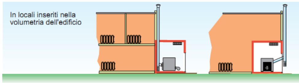
Figura 14 – Luoghi di installazione degli apparecchi
