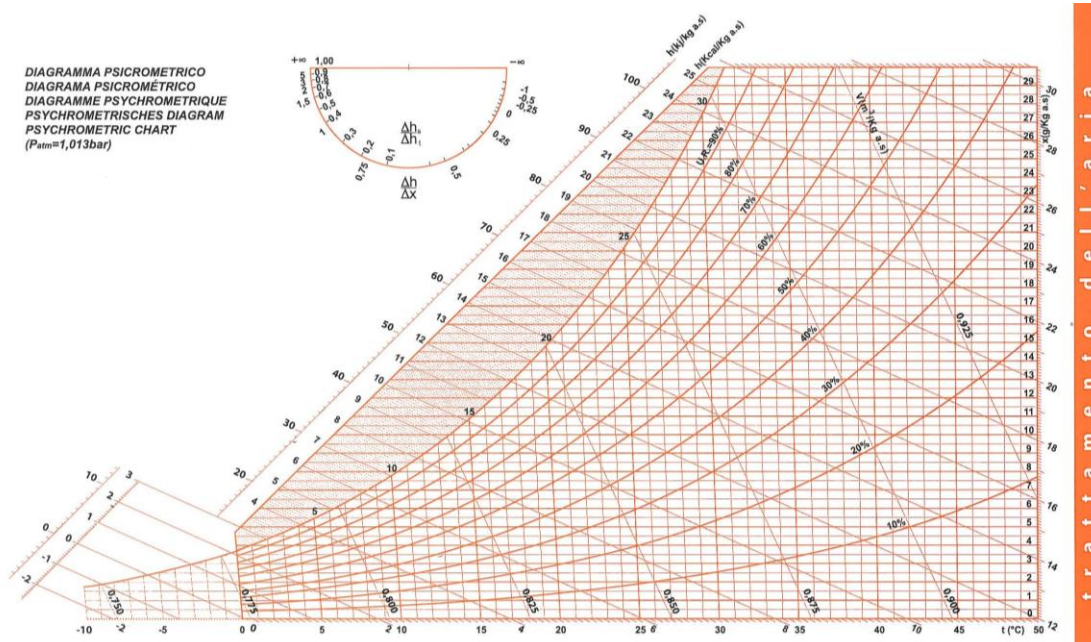
Figura 1 - Diagramma psicrometrico
