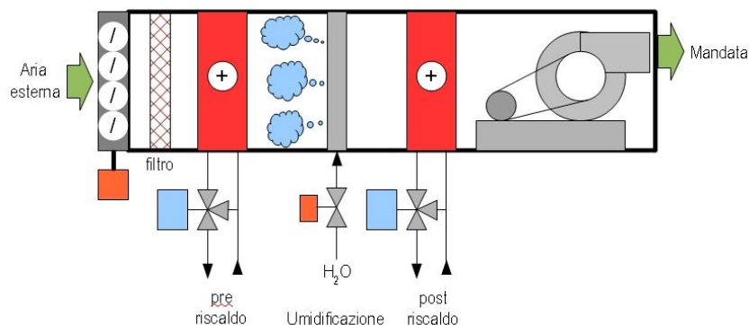
Figura 58 - Una c.t.a. con solo aria esterna: è detta anche ad "aria primaria"
