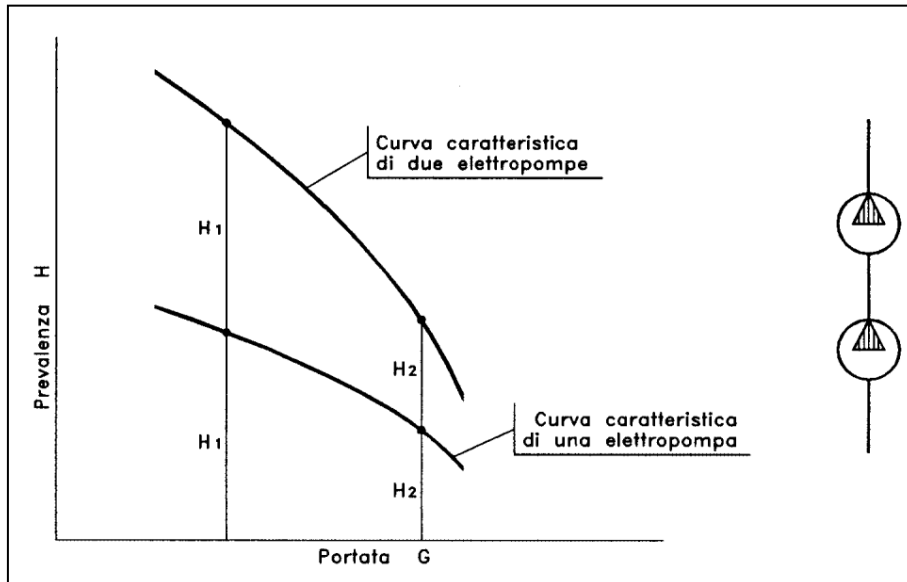
Figura 90 - Elettropompe montate in serie
