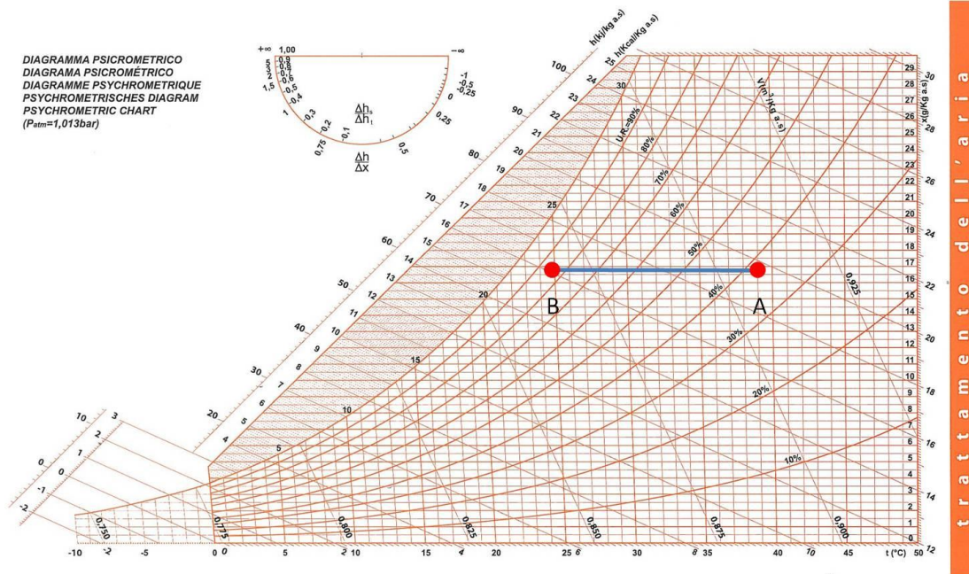
Figura 65 - Raffreddamento senza deumidificazione (dal punto A al punto B)
