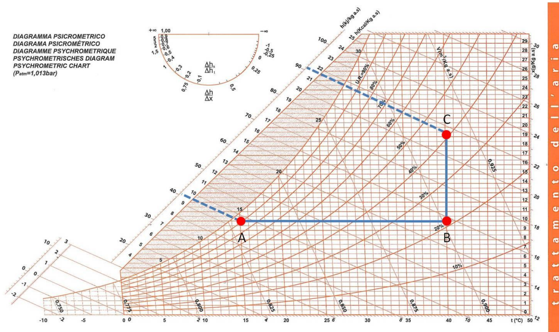
Figura 7 – Riscaldamento sensibile + latente (dal punto A al punto C)
