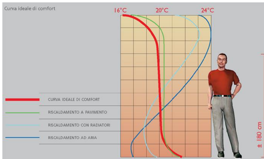
Figura 48 - Curva termica
