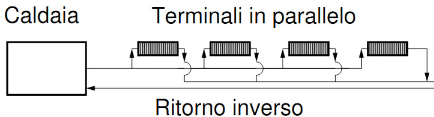
Figura 29 - Distribuzione a due tubi con ritorno inverso
