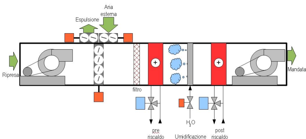
Figura 60 - una c.t.a. con tre serrande: aria esterna/espulsione/miscela
