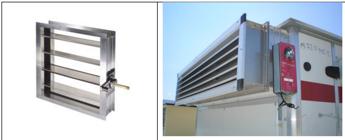
Figura 57 - Come è fatta una serranda e il suo posizionamento
