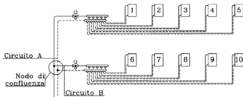
Figura 31 - Distribuzione con collettori Modul
