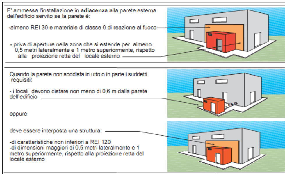
Figura 15 –Installazione in locali esterni
