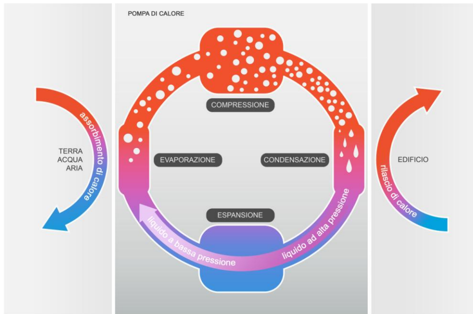
Figura 20 - Schema del ciclo di una pompa di calore
