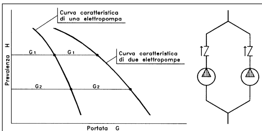
Figura 91 - Elettropompe montate in parallelo
