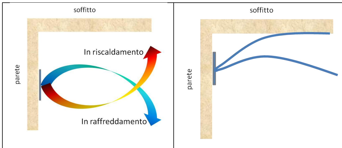
Figura 74 – Getto senza effetto Coanda (sinistra) e con effetto Coanda (a destra)
