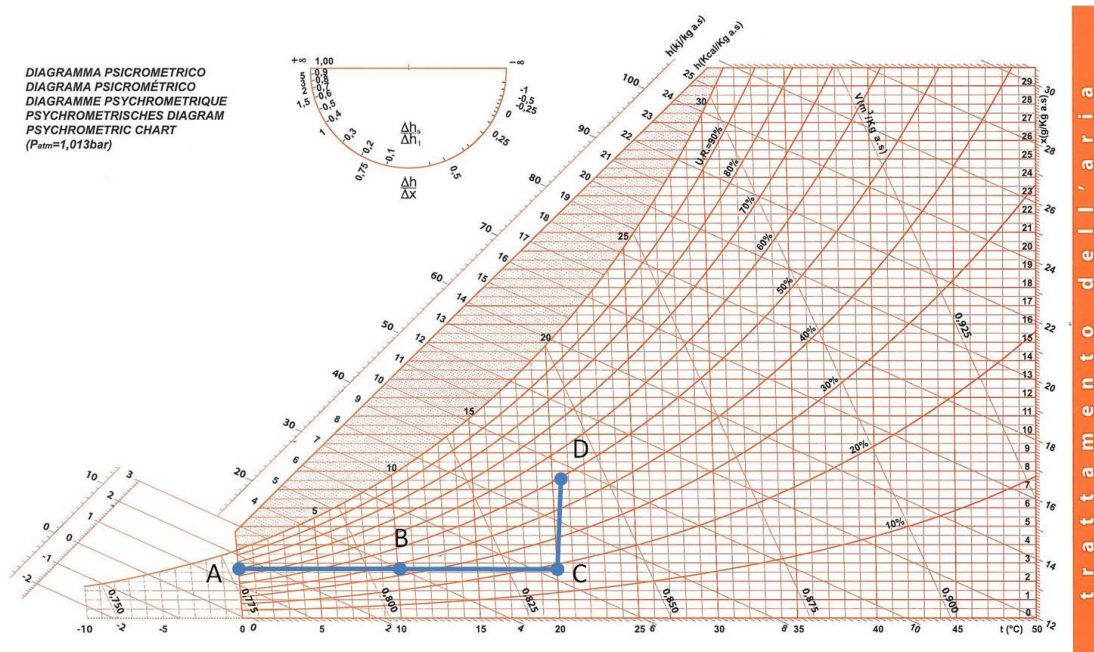
Figura 96 - Trattamenti termici invernali nella u.t.a.
