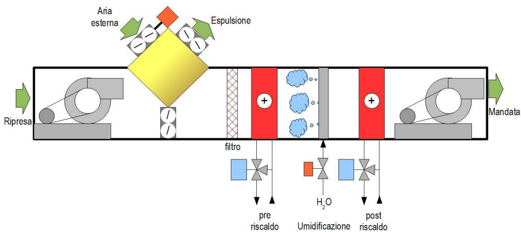
Figura 62 - Una c.t.a. aria primaria con recuperatore
