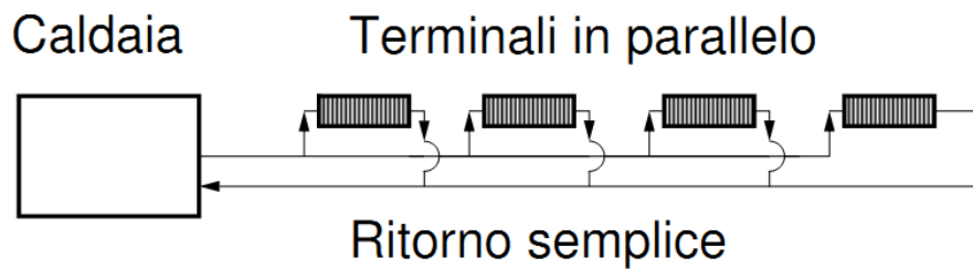
Figura 28 - Distribuzione a due tubi con ritorno semplice
