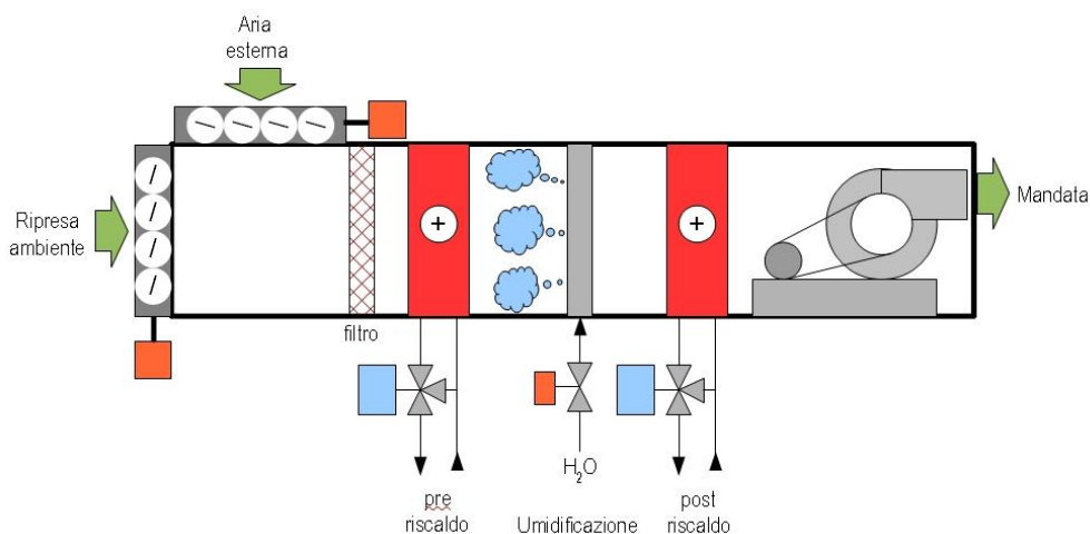
Figura 59 - una c.t.a. con recupero ambiente e aria esterna
