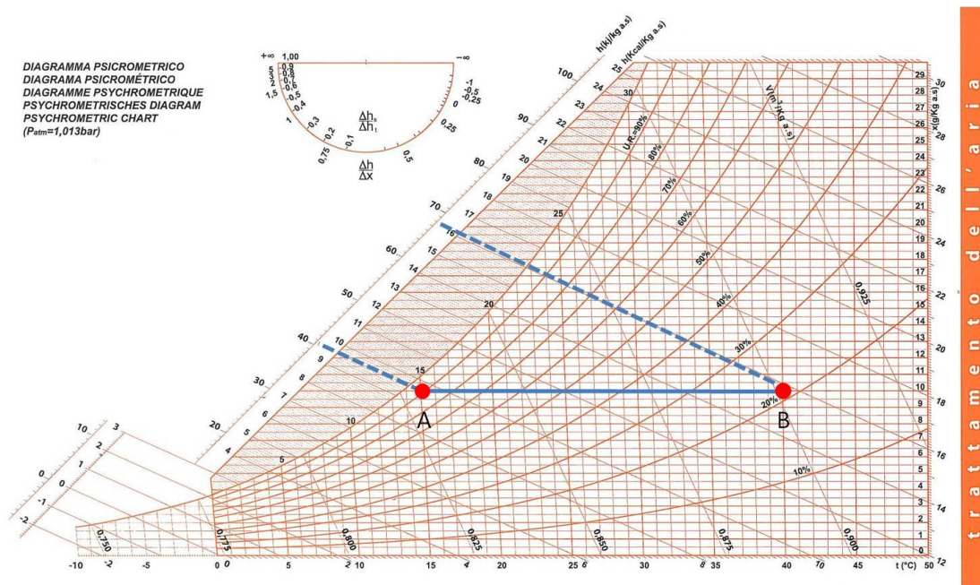
Figura 5 – Riscaldamento sensibile (dal punto A al punto B)
