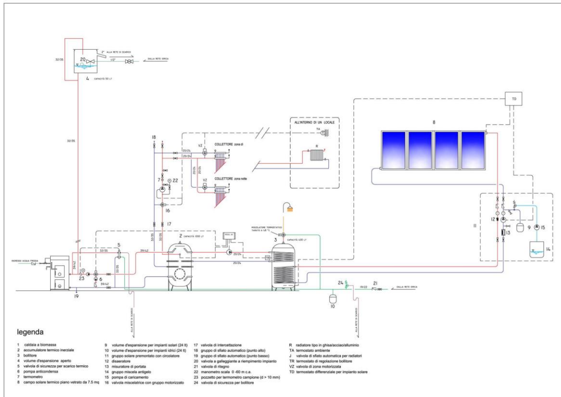
Figura 97 – Esempio di schema funzionale di centrale termica
