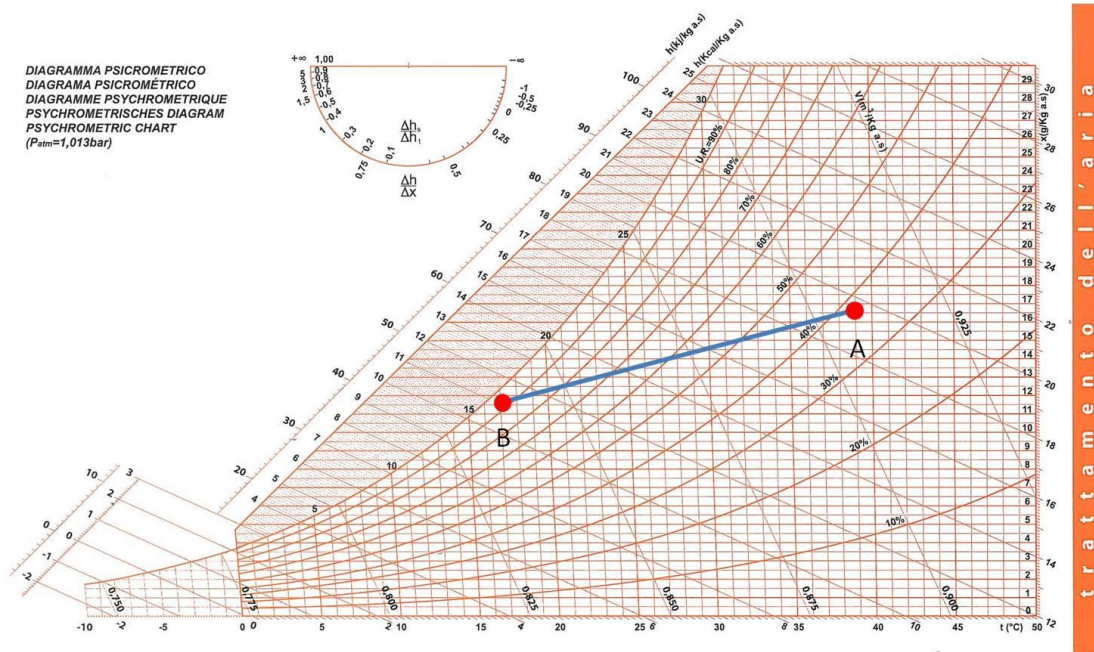
Figura 66 – Raffreddamento con deumidificazione (dal punto A al punto B)
