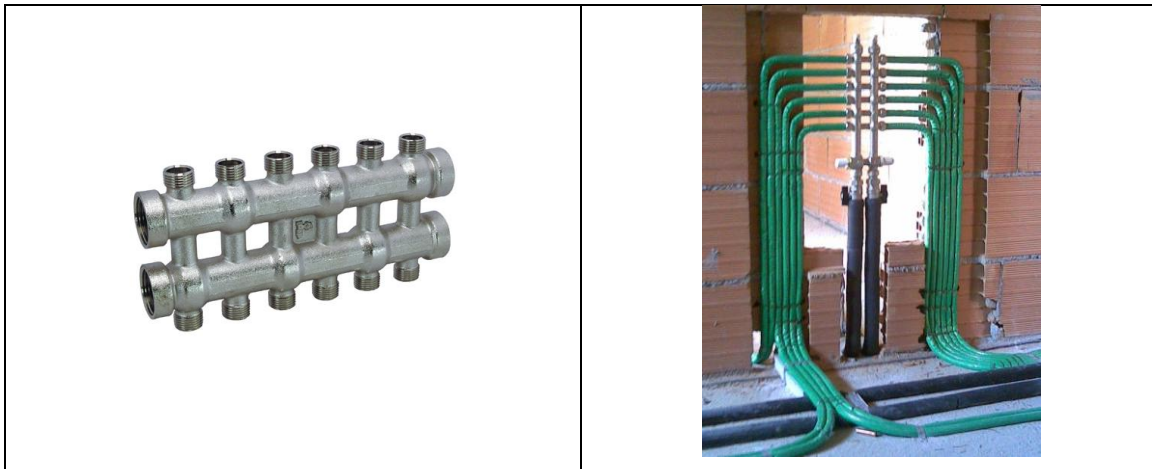
Figura 30 - Collettore modul a sei attacchi (a sinistra) e montato (a destra)
