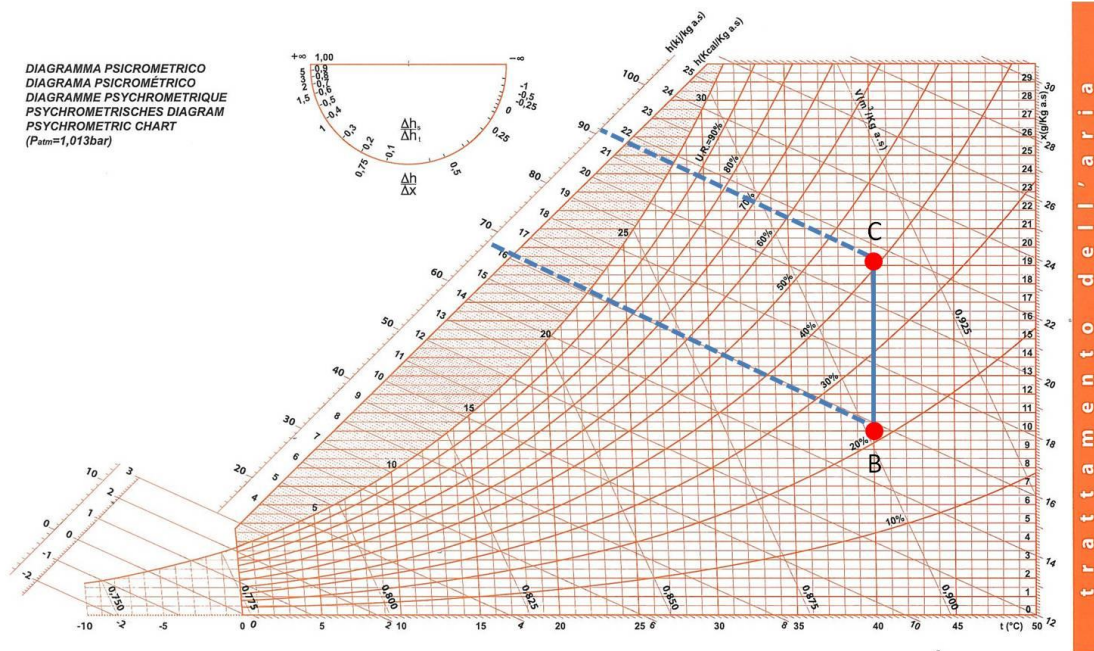
Figura 6 - Riscaldamento latente (dal punto B al punto C)
