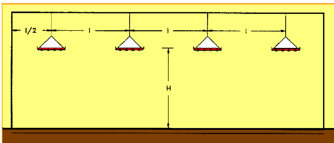
Figura 52 – Rapporto tra la distanza di installazione e l'altezza di installazione
