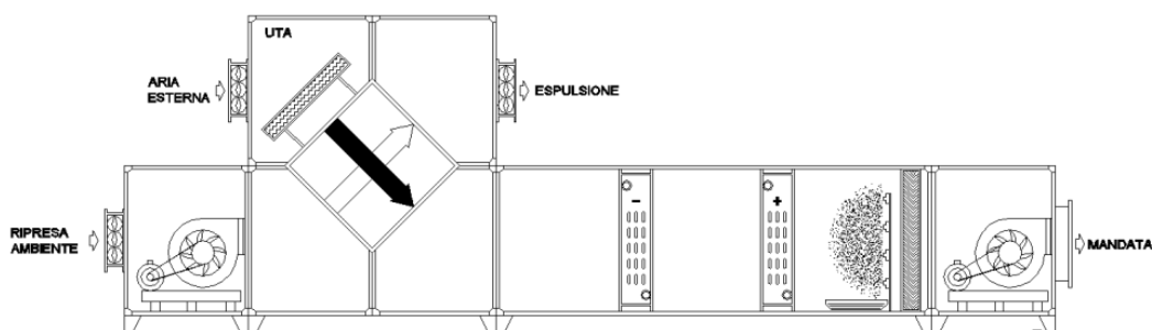
Figura 95 - Schema funzionale della centrale di trattamento aria di progetto
