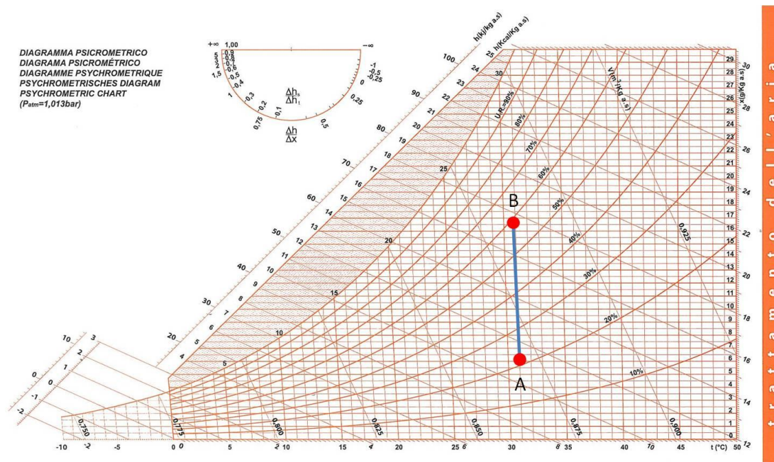
Figura 68 - Umidificazione a vapore (dal punto A al punto B)
