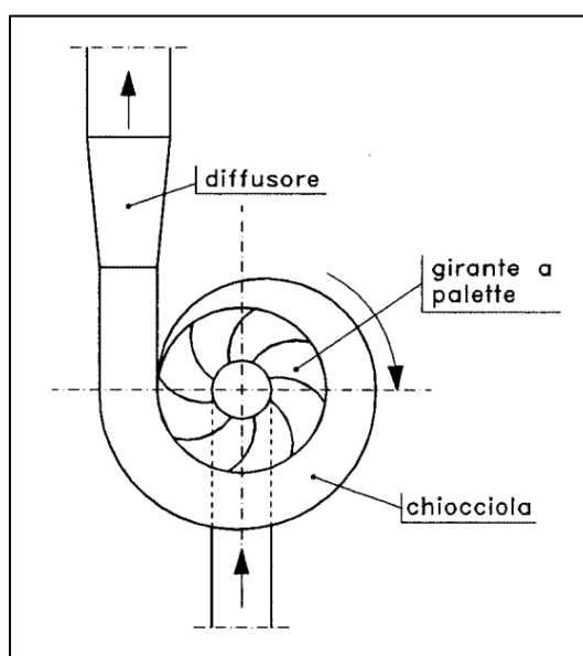
Figura 87 - Schema funzionale di una pompa centrifuga
