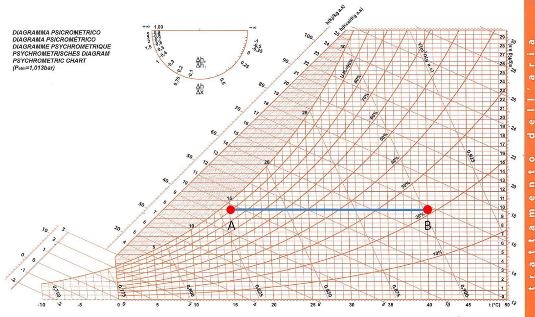
Figura 64 - Riscaldamento (dal punto A al punto B)
