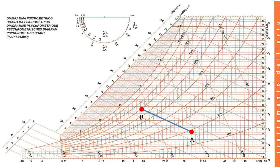
Figura 67 - Umidificazione adiabatica (dal punto A al punto B)
